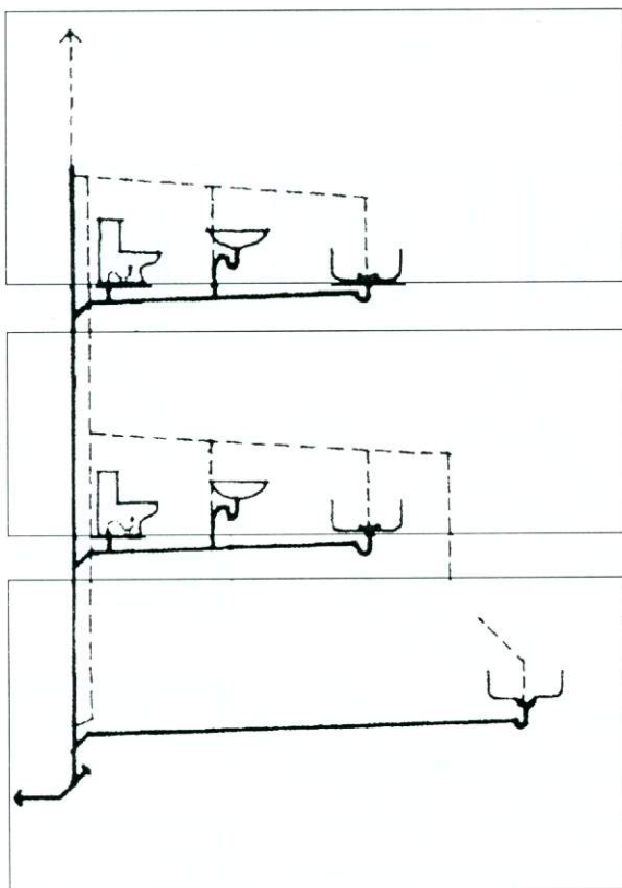
Hệ thống thoát nước
