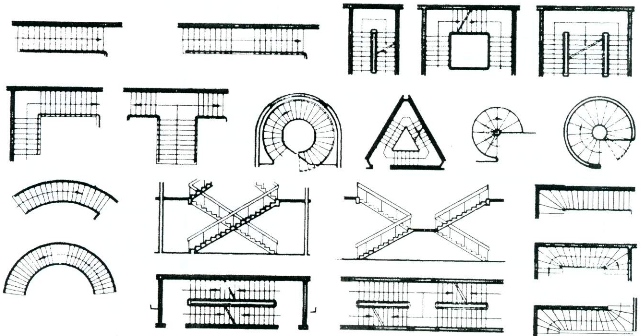
Hình thức mặt bằng của cầu thang
