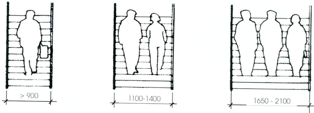
Độ rộng của cầu thang.
